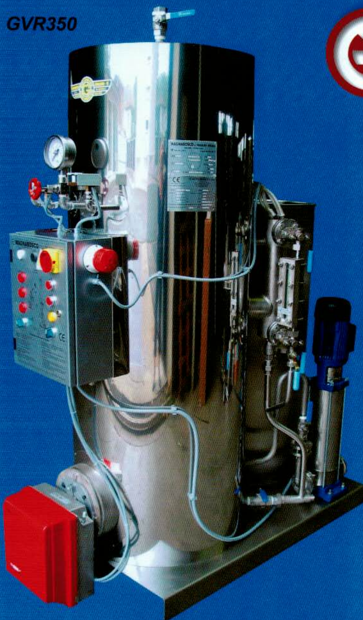
Generatore di vapore in acciaio inox tipo GVR 350 Stainless steel steam boiler type GVR 350
